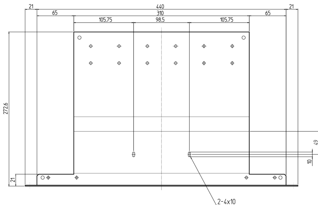
【上面】
