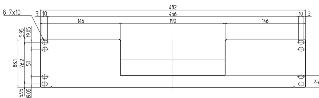
【前面】
